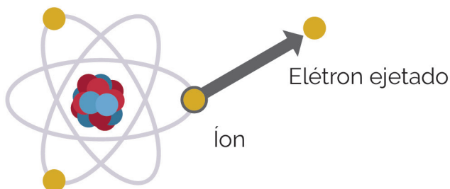
Figura 2 - Processo de ionização.
