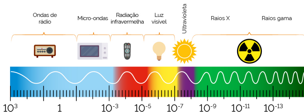
Figura 1 - Espectro das ondas eletromagnéticas
