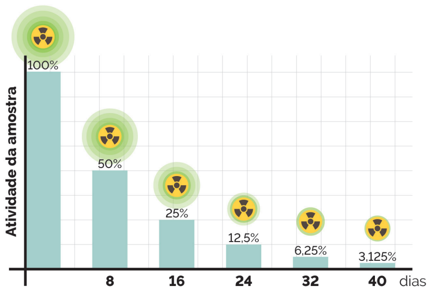
Figura 5 - Decaimento do ^{131}\text{I} pela sua meia-vida física de 8 dias.
