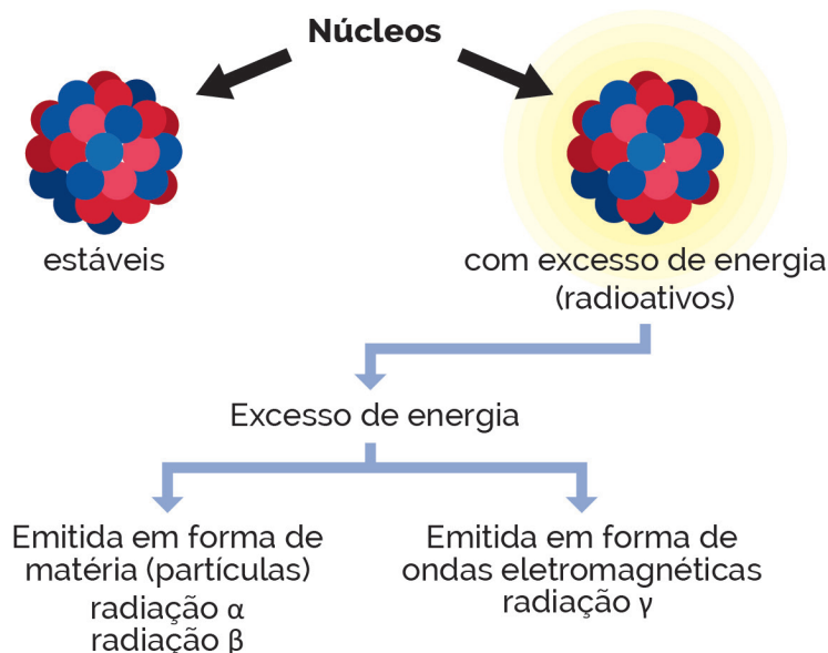
Figura 4 - Processo de desintegração do radionuclídeo.
