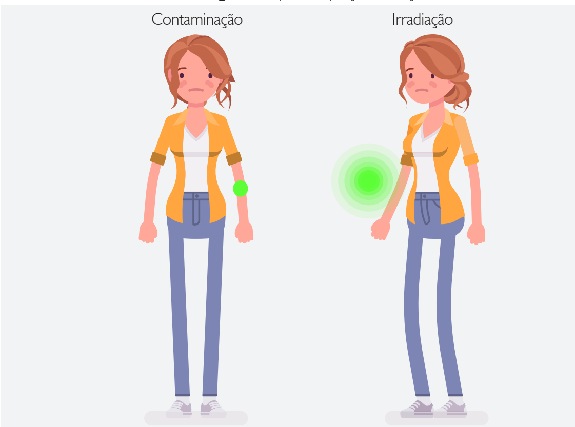
Figura 7 - Tipos de exposição à radiação.
